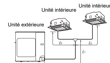
Figure de l'installation double simultanée
